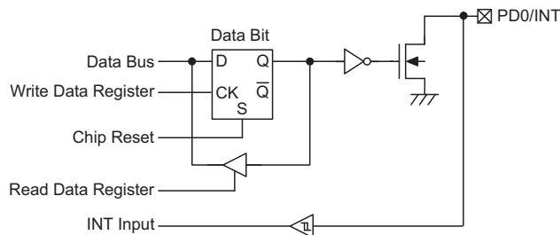
PD0 Input/Output Port
