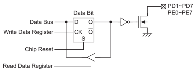
PD1~PD7, PE Output Ports
